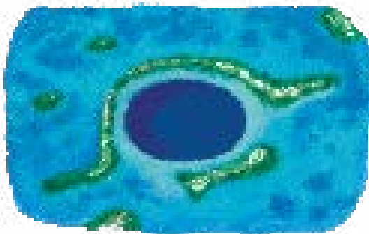
la dolina marina
